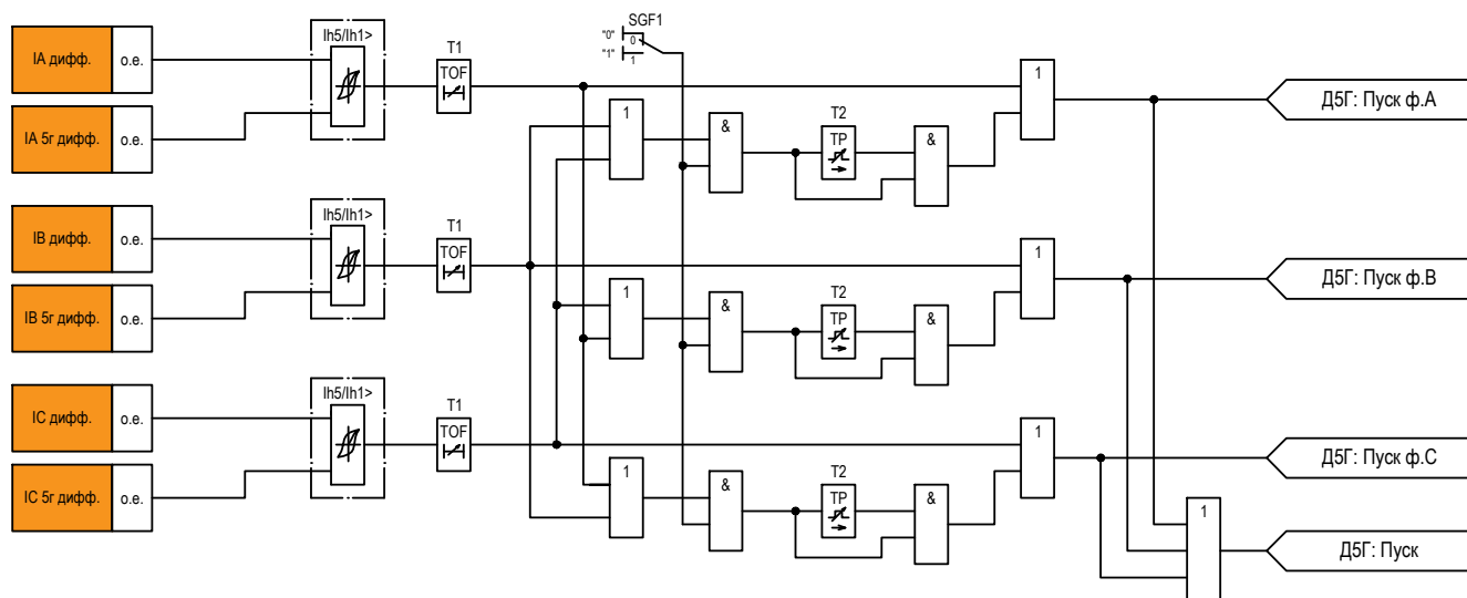
Рисунок 2.6 – Функциональная схема «Д5Г»
